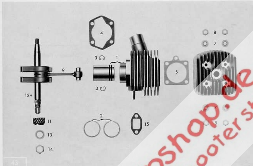
Tafel 5 Zylinder – Kurbeltrieb
