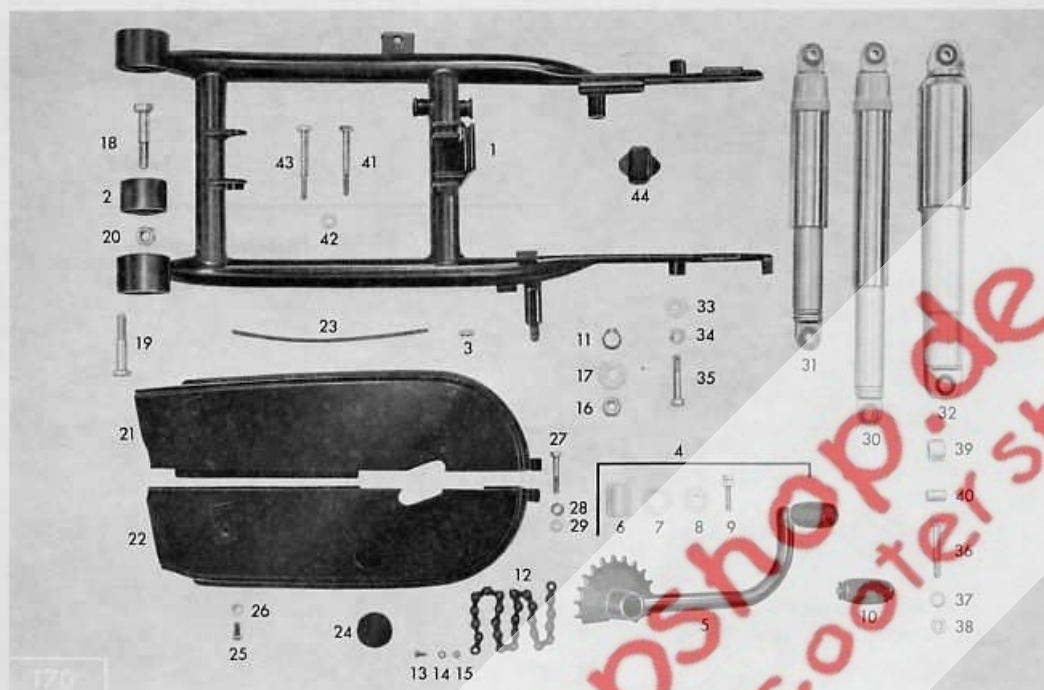
Tafel 3 Hinterradschwinge – Kickstarter – Kettenkasten – Federbein
